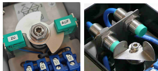
Pepperl+Fuchs links: 2x verstellbare Aluminium-Schaltfahne, rechts: 1x Edelstahl-Schaltfahne 0° und 90°.
